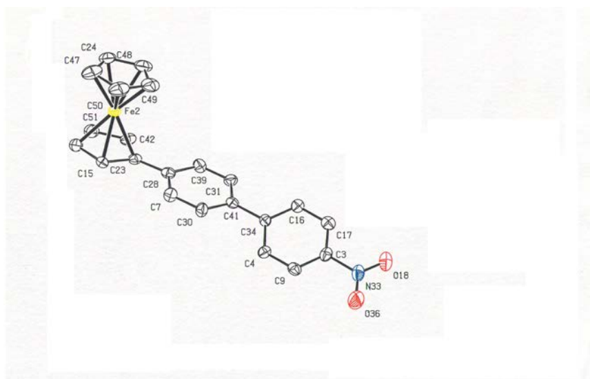
Obr. 1 Krystalová struktura 4-nitrobifenylferrocenu
